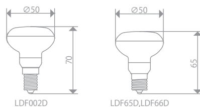
寸法図
