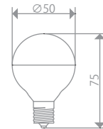
LDF92,71
