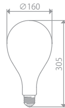
LDF302
