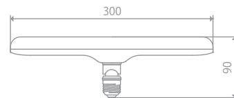
LDC5
