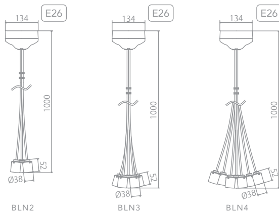
BLN2
