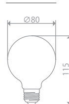
寸法図
