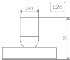
SLB2
