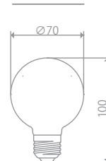
寸法図
