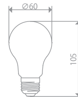
寸法図
