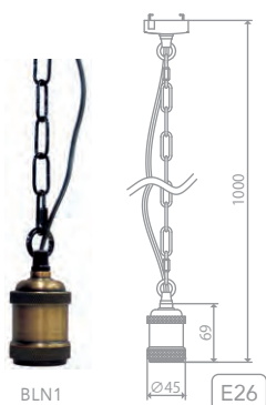
BLN1
