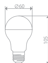
寸法図
