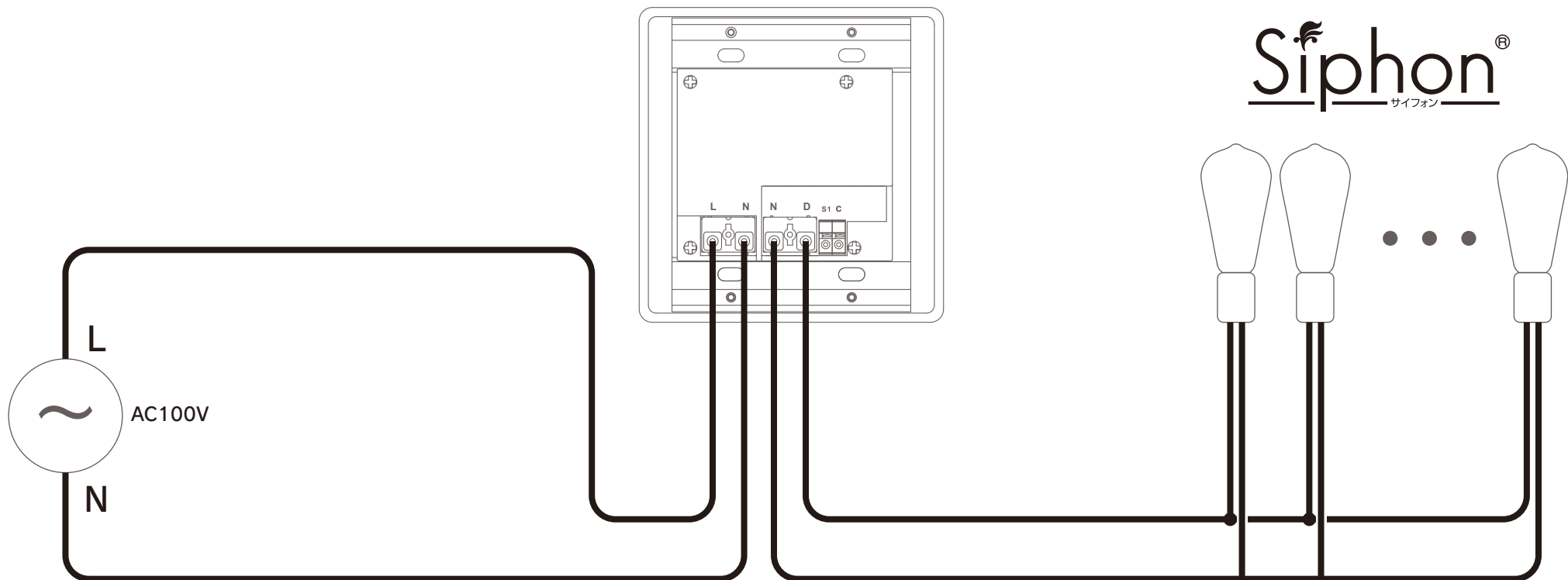
位相制御式調光器 ファースト・デザイン・システム製 FLC-800D 使用例
